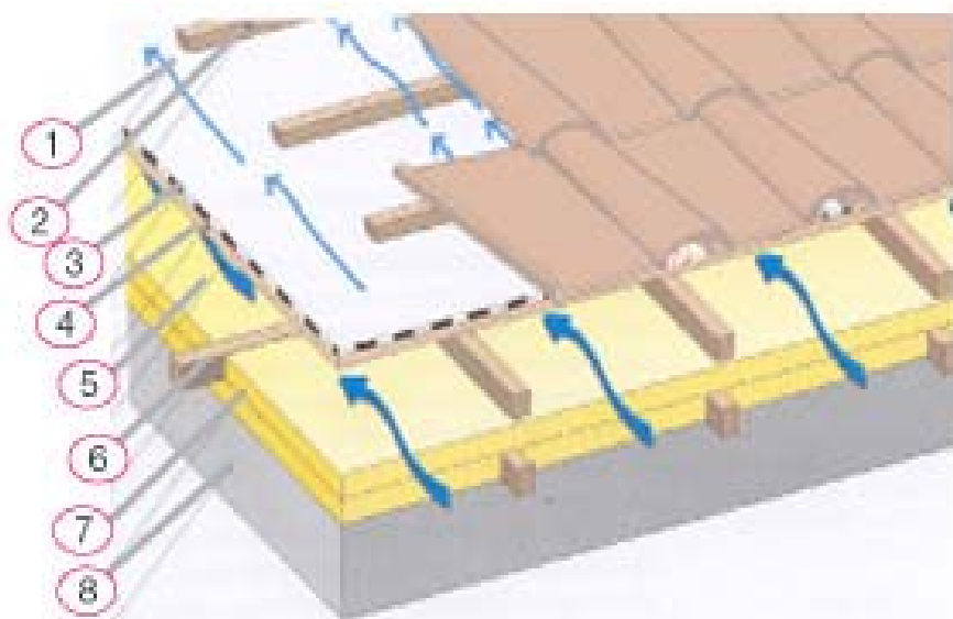
Fig.3 Intercapedine doppia
