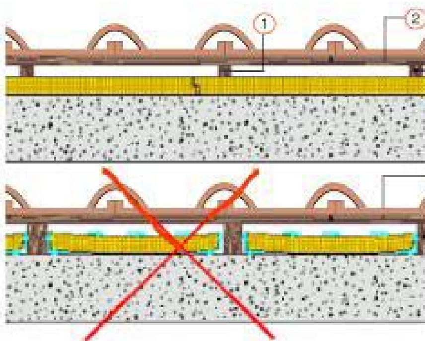
Fig.6 Strato Termoisolante
