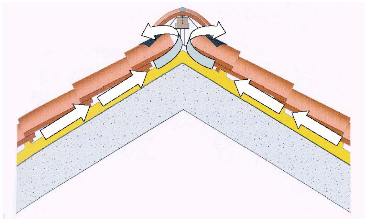
Fig. 1 Moto convettivo dell'aria
